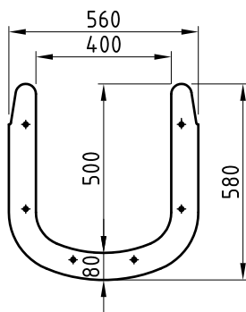
einstieg [ansicht A] m=1:20
