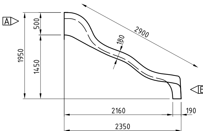
[schnitt 1-1] m=1:50
