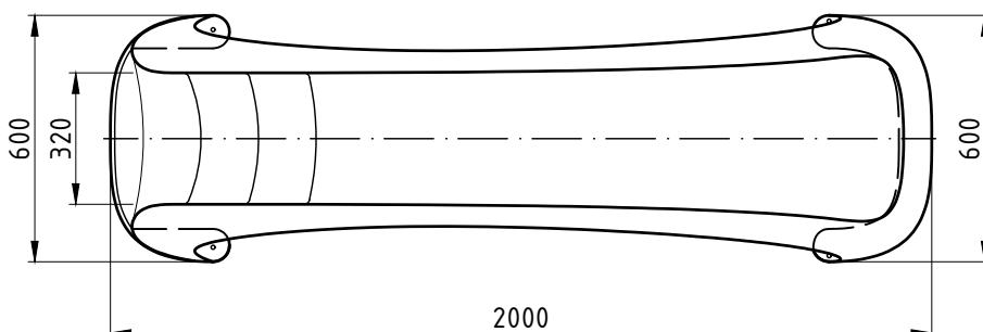
[grundriss] m=1:20
