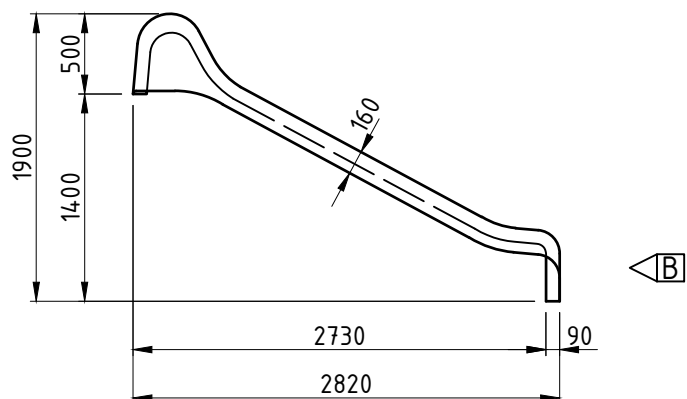
[schnitt 1-1] m=1:50
