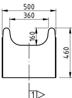
ausstieg [ansicht B] m=1:20
