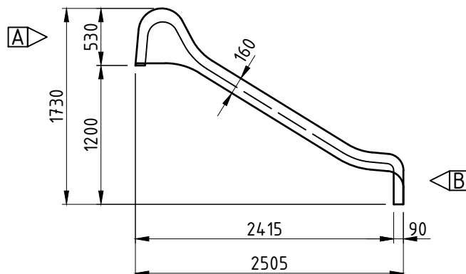
[schnitt 1-1] m=1:50
