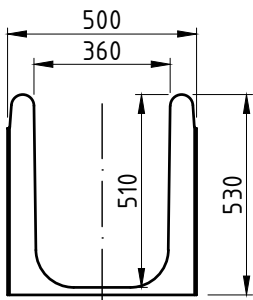
einstieg [ansicht A] m=1:20
