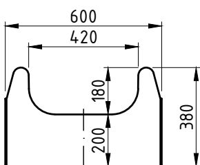
ausstieg [ansicht B] m=1:20
