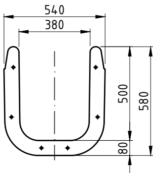
1 einstieg [ansicht A] m=1:20
